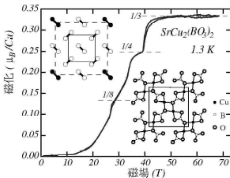
図4 0.08 Kで測定した \text{SrCu}_2(\text{BO}_3)_2 の磁化曲線。 \text{Cu}^{2+} の飽和磁化の 1/3 , 1/4 , 1/8 の磁化にプラトーが存在する。挿入図右は [001] 方向からみた \text{SrCu}_2(\text{BO}_3)_2 の結晶構造 ( \text{CuBO}_3 面)。挿入図左は 1/8 プラトーが観測された当時，提案された超格子構造 (図5の超格子と比較されたい)。白ダンベルと黒ダンベルは，それぞれスピン一重項状態とスピン三重項状態。実線は結晶構造の単位格子で点線は磁気構造の単位格子。
