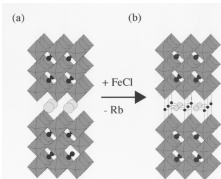
図6 \text{RbCa}_2\text{Ta}_3\text{O}_{10} (左) と (\text{FeCl})\text{Ca}_2\text{Ta}_3\text{O}_{10} (右)
