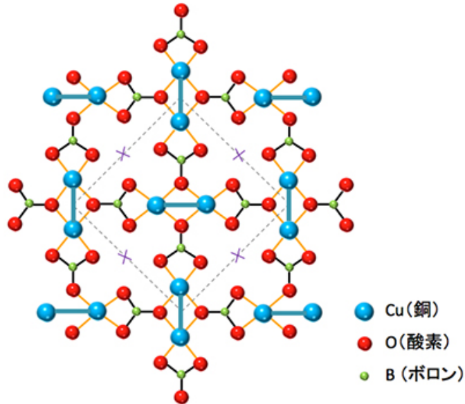
図2： \text{SrCu}_2(\text{BO}_3)_2 の結晶における \text{CuBO}_3 二次元平面の模式図。Cuイオンは図の青線で模式的に示したように、電子スピン対（ダイマー）をつくる。
