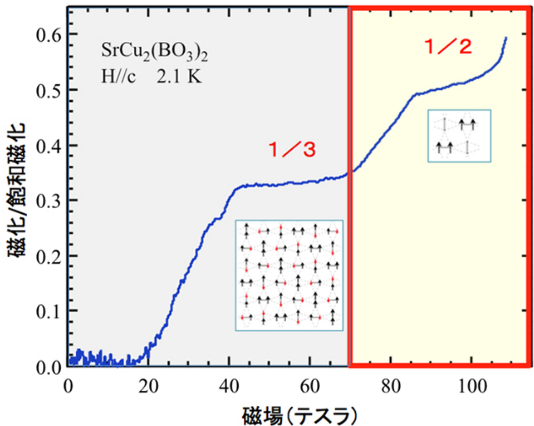
図3：SrCu 2 (BO 3 ) 2 の磁化過程。赤線で囲った黄色の部分今回新しく観測できた領域。2分の1量子状態のプラトーの長さは3分の1プラトーの7割程度であり、完全に平坦にもなっていないことから2分の1プラトーの安定性は3分の1プラトーのものより弱いことがわかる。
